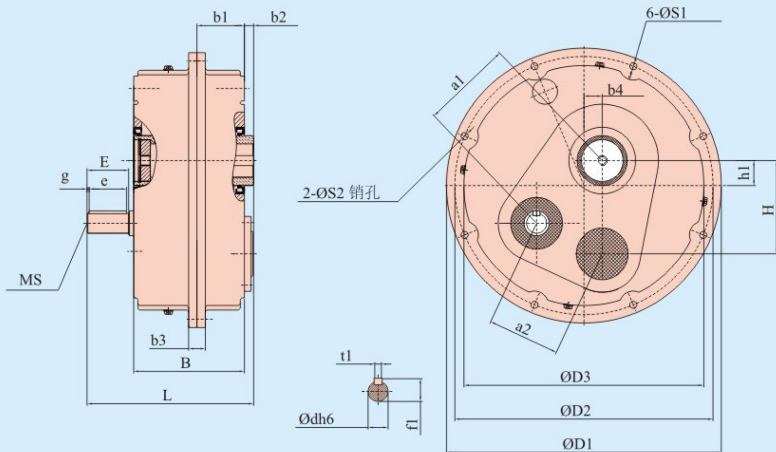
XG35- XG125 的外形尺寸
